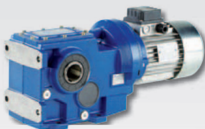
Коническоцилиндрические мотор-редукторы Helical bevel geared motors
